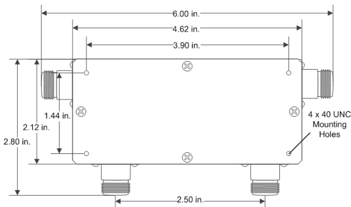
W8540 Circulator Dimensions
